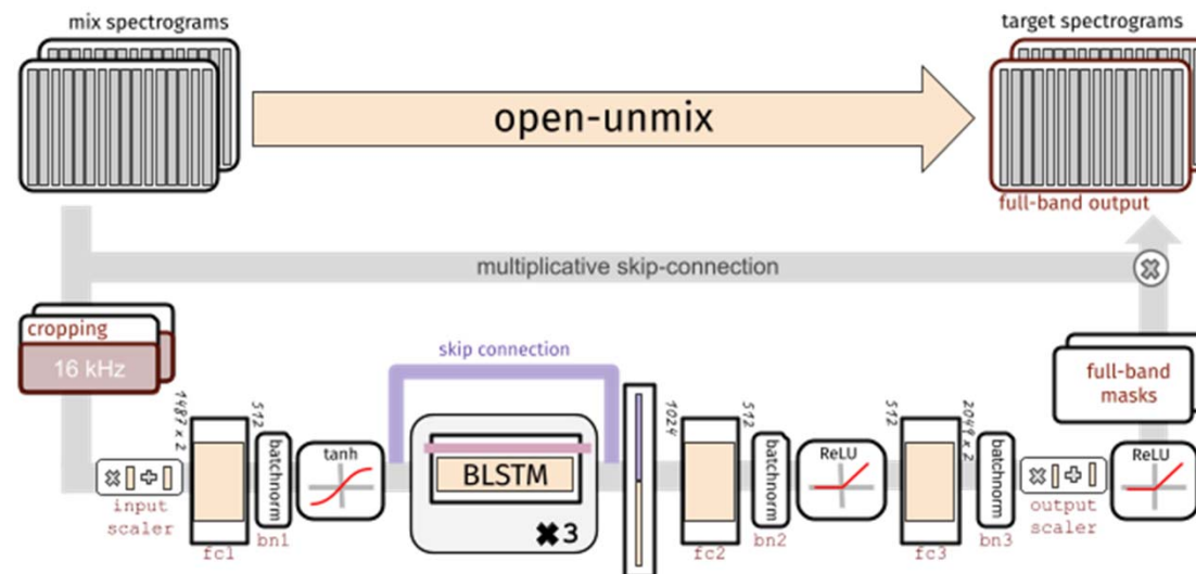
図2 Open-Unmix のアーキテクチャ
