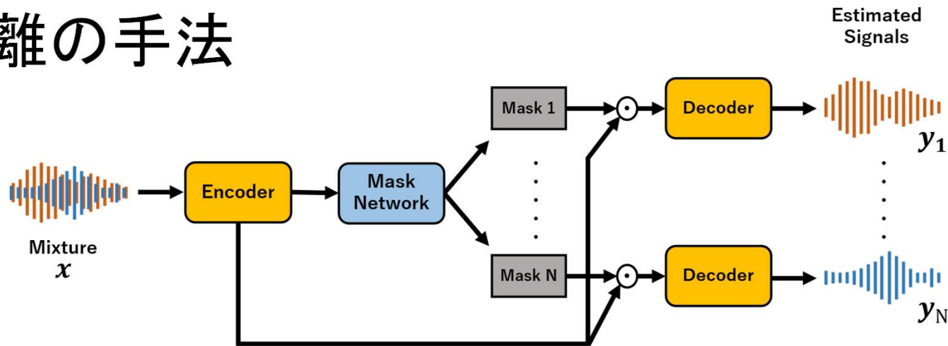
図1 マスク推定による音源分離
